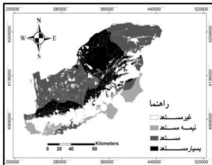
شکل ۷- استعداد سنگی اراضی کشاورزی جهت کشت سویا برای عوامل اقلیمی در استان گلستان
