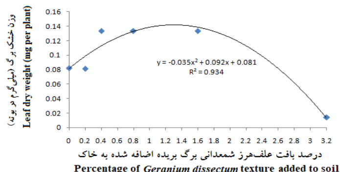
شکل ۵- برازش مدل پتانسیل آلوپاتیک درصد بافت علف‌هرز شمعدانی برگ بریده اضافه شده به خاک بر وزن خشک برگ در بوته کلزا
