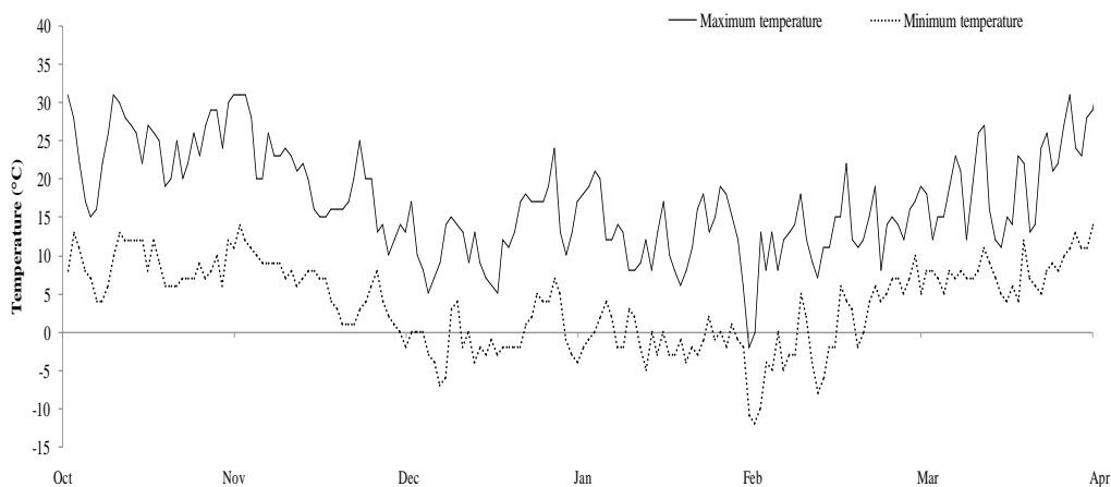
شکل ۱- حداقل و حداکثر درجه حرارت روزانه مشهد طی فصل رشد عدس در سال ۱۳۹۶ Figure 1- Daily minimum and maximum temperature during 2017 lentil growing season, Mashhad
