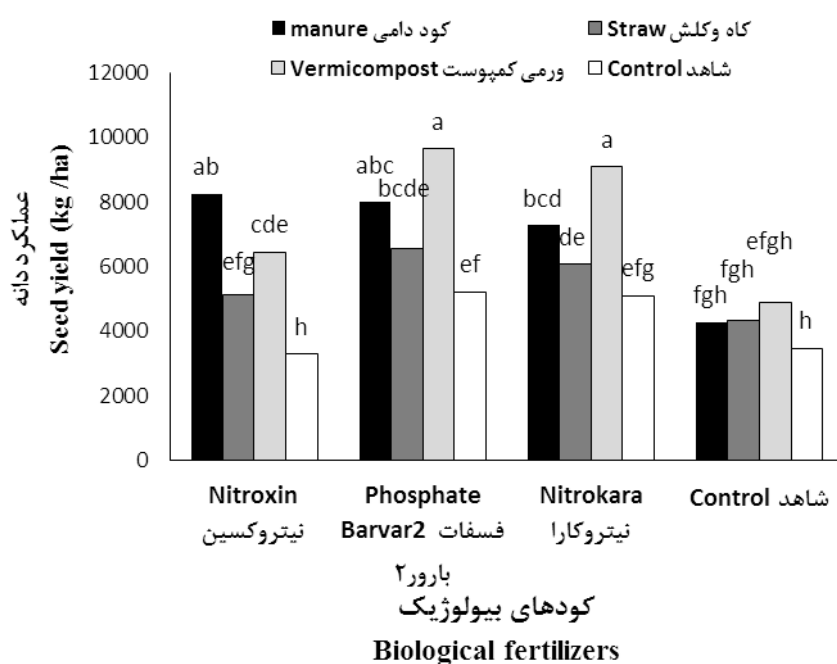
شکل ۲- اثر متقابل کودهای آلی و زیستی بر عملکرد دانه گیاه ذرت
