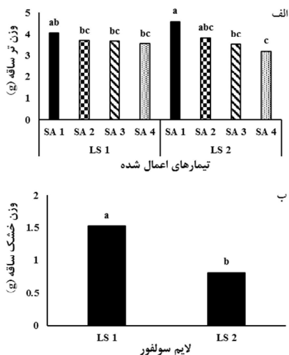
شکل ۴- الف) اثر تیمارهای اعمال شده بر وزن تر ساقه و ب) وزن خشک ساقه، LS1= لایم سولفور صفر درصد LS2= لایم سولفور پنج درصد SA1= سالیسیلیک اسید صفر مولار SA2= سالیسیلیک اسید 10^{-6} مولار SA3= سالیسیلیک اسید 10^{-4} مولار SA4= سالیسیلیک اسید 10^{-2} مولار * ستون‌های دارای حرف مشترک اختلاف معنی‌دار ندارند.
